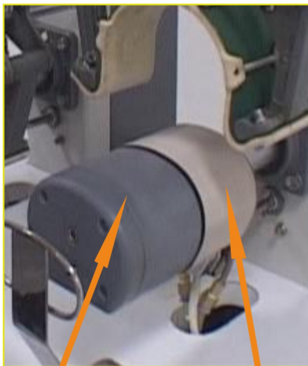
冷卻模 Cooling
