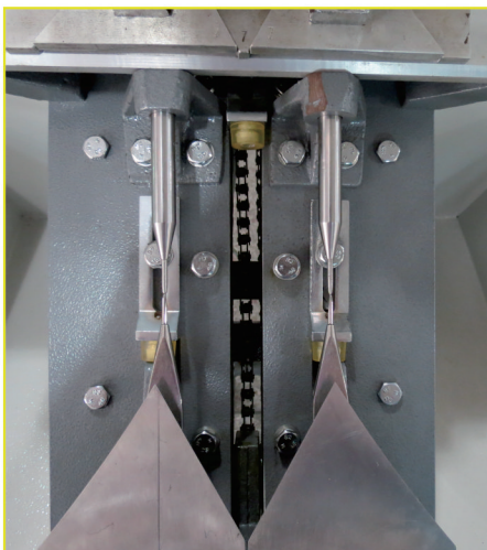
撞針 Striker
