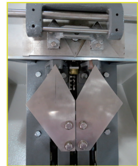
CF-44 反領機 Collar mould
