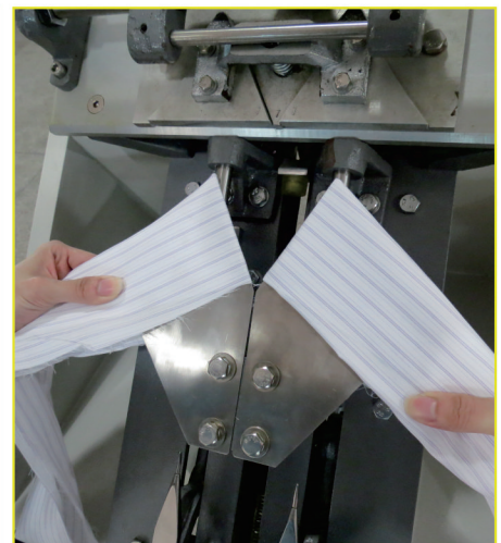
壓燙 Press
